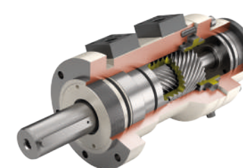
HYDRAULISKA VRIDDON
