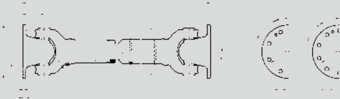
Normalausführung - größerer Flansch Standard design - large flange diameter
